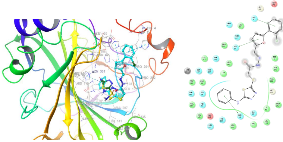
Şekil 2.2. Asetazolamit ve 1 nolu bileşiğin hCA II enzimi üzerindeki docking pozisyonları ve amino asit etkileşimleri (1 nolu bileşik siyan mavimsi, asetazolamit de koyu yeşil renklerle gösterilmiştir. Yeşil çizgiler \pi - \pi bağları ve çinko atomu gri küre olarak belirtilmiştir.)
