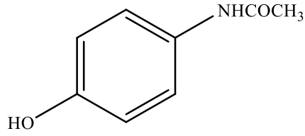
Şekil 2.3. Parasetamolün kimyasal formülü
